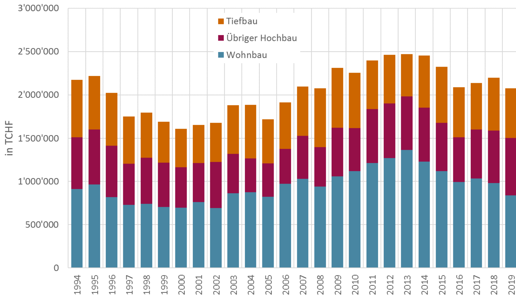
Bauinvestitionen Graubünden
